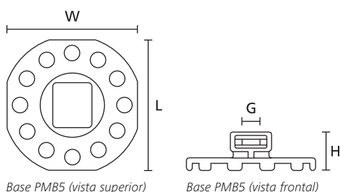
Base PMB5 (vista superior)
