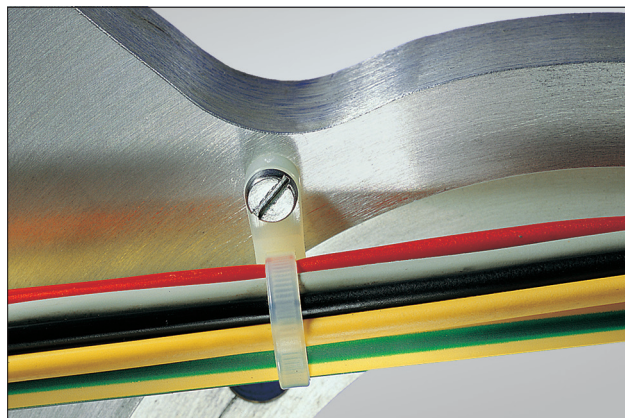
As abraçadeiras com cabeça para fixação são facilmente parafusadas no painel.
