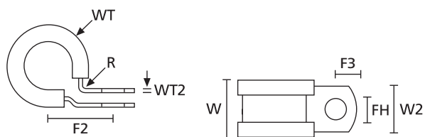
ALU-C (vista lateral)
