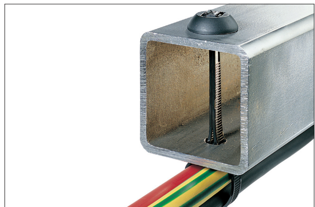
Montagem simples da abraçadeira graças ao serrilhado em ambos os lados.
