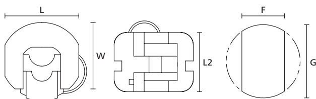
Prensa cabos, série PC
