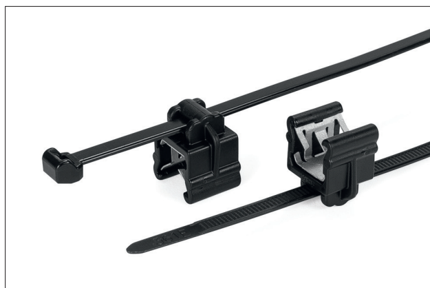
Abraçadeira com clip de fixação EC.
